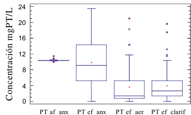
Figura 8. Comportamiento de P en el tren II
