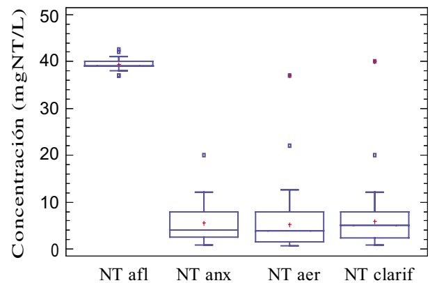
Figura 6. Eliminación de nitrógeno total en tren II
