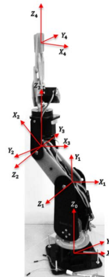
Figura 2. Modelo esquemático de las juntas del manipulador de 4 DOF
