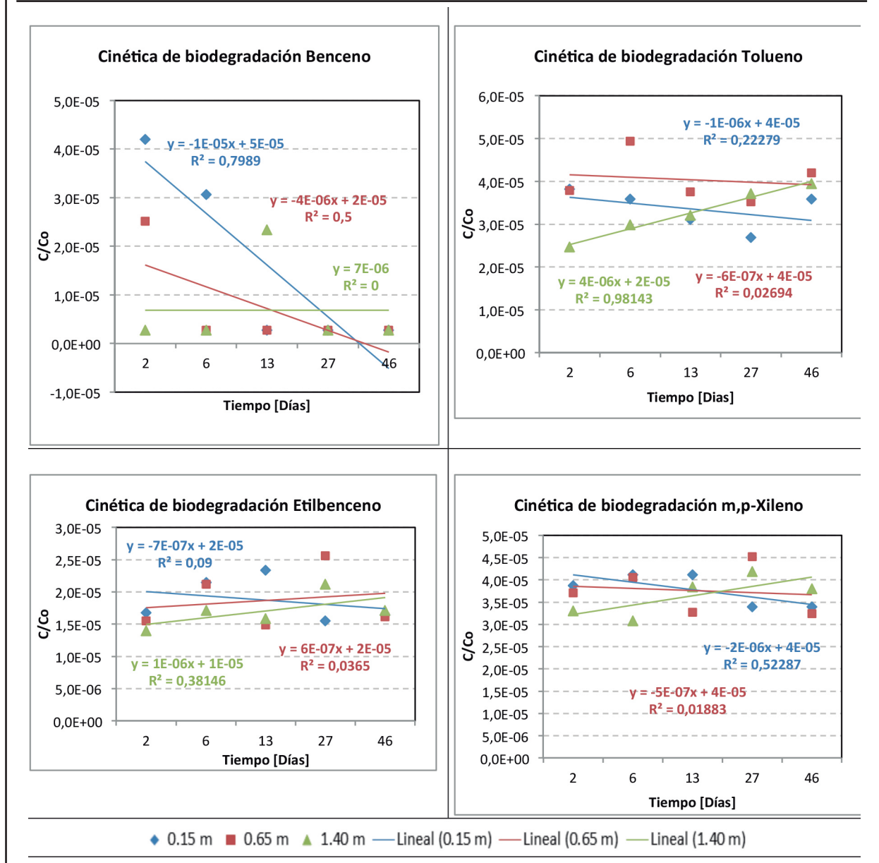
Figura 8. Cinéticas de biodegradación de los componentes de la gasolina E10
