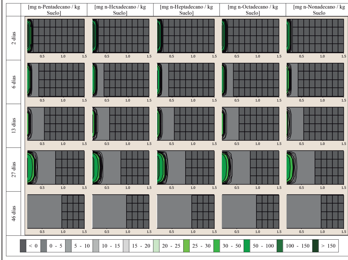
Figura 12. Distribución de concentración a través del tiempo de los componentes de la Diesel B10 durante el proceso de biorremediación. (Cont).
