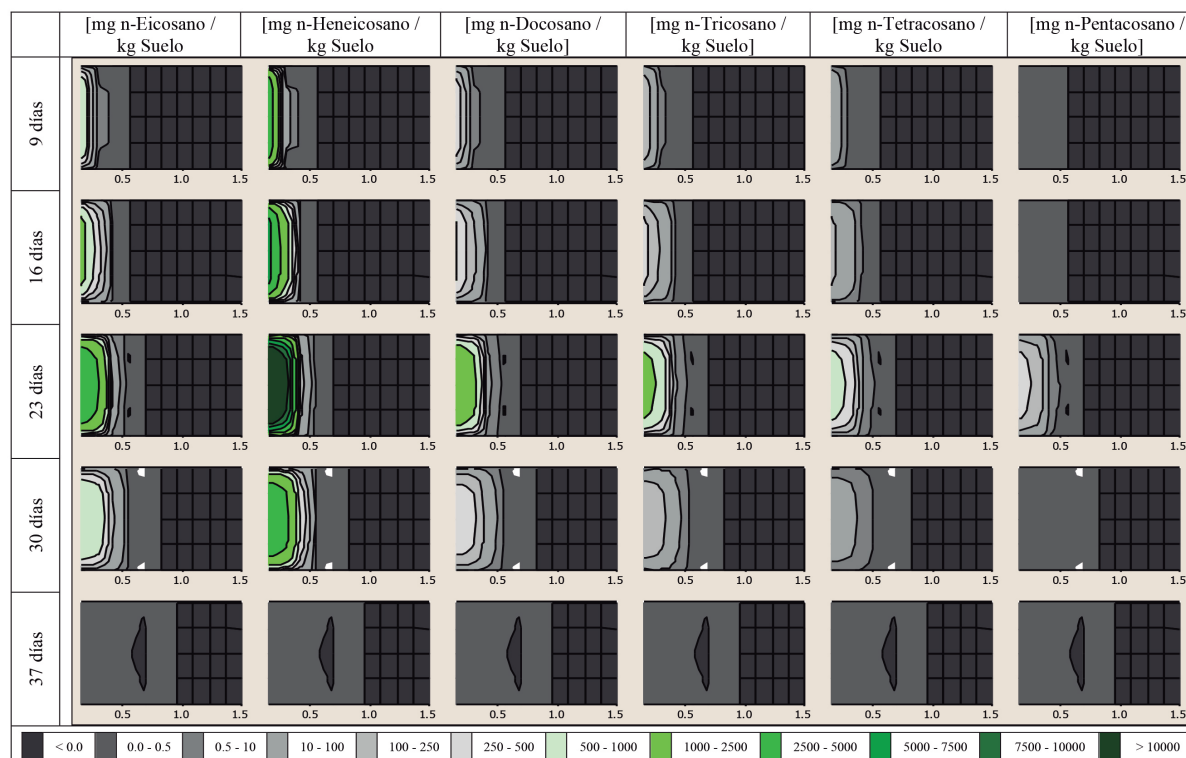
Figura 18. Comportamiento dinámico de los componentes de la Diesel B10 a través del tiempo en el suelo. (Cont.)
