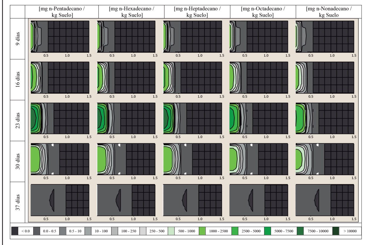
Figura 17. Comportamiento dinámico de los componentes de la Diesel B10 a través del tiempo en el suelo (Cont.)
