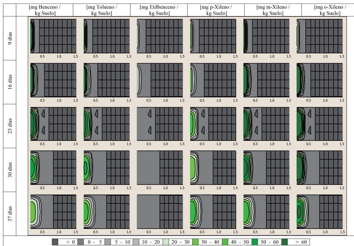
Figura 14. Comportamiento dinámico de los componentes de la Gasolina E10 a través del tiempo en el suelo
