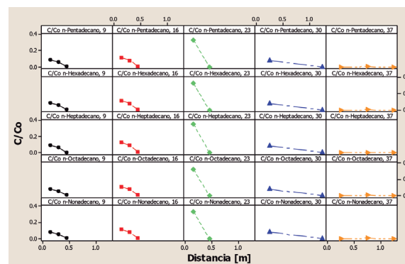
Figura 20. Distribución de concentración de compuestos del Diesel B10 en el tiempo. (Cont.)
