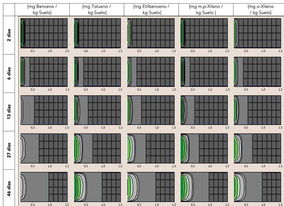
Figura 10. Distribución de concentración a través del tiempo de los componentes de la Gasolina E10 durante el proceso de biorremediación
