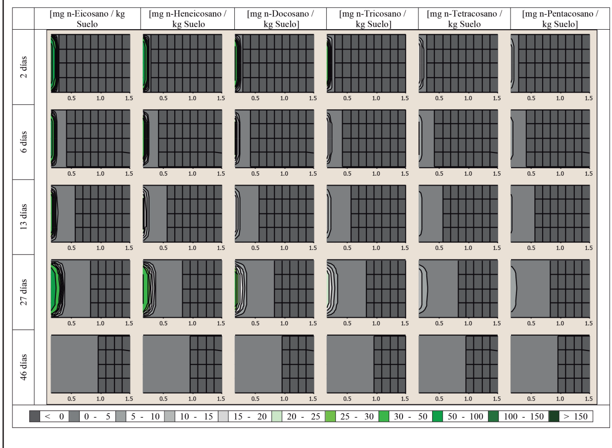
Figura 13. Distribución de concentración a través del tiempo de los componentes de la Diesel B10 durante el proceso de biorremediación. (Cont.)
