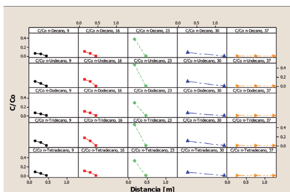
Figura 19. Distribución de concentración de compuestos del Diesel B10 en el tiempo
