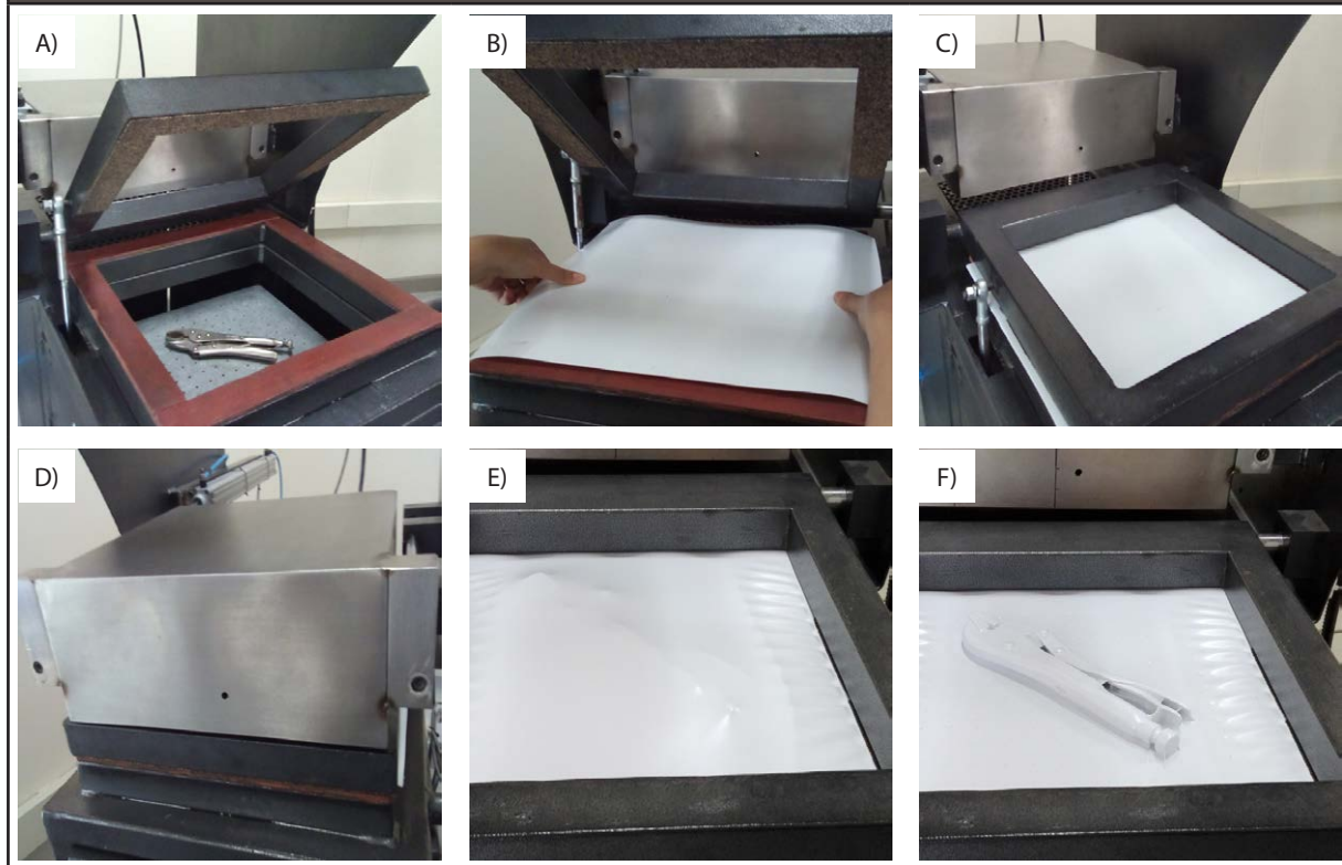
Figura 12. Puesta a punto maquina automatizada de termoformado, a) posicionamiento del molde, b) ubicación de lámina, c) sujeción lamina, d) etapa de calentamiento, e) elevación del molde contra la lámina y f) accionamiento de vacío y motor ventilador.
