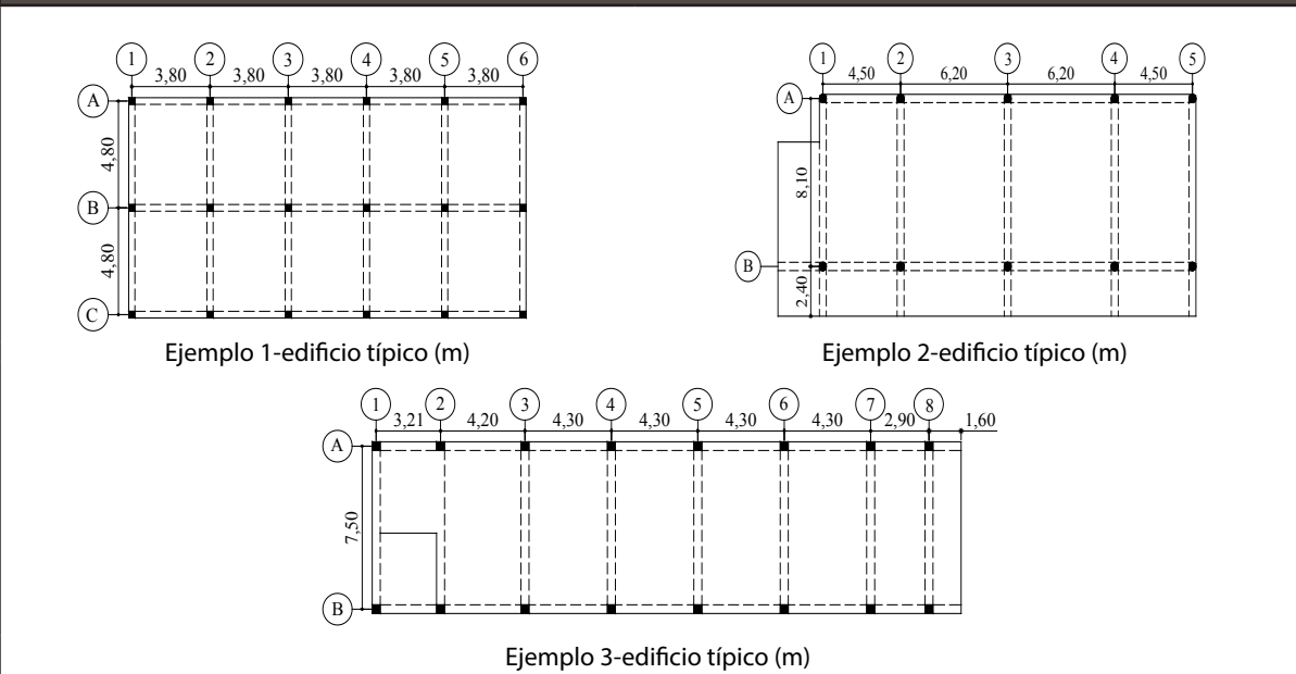
Figura 3. Configuración estructural típica de las escuelas
