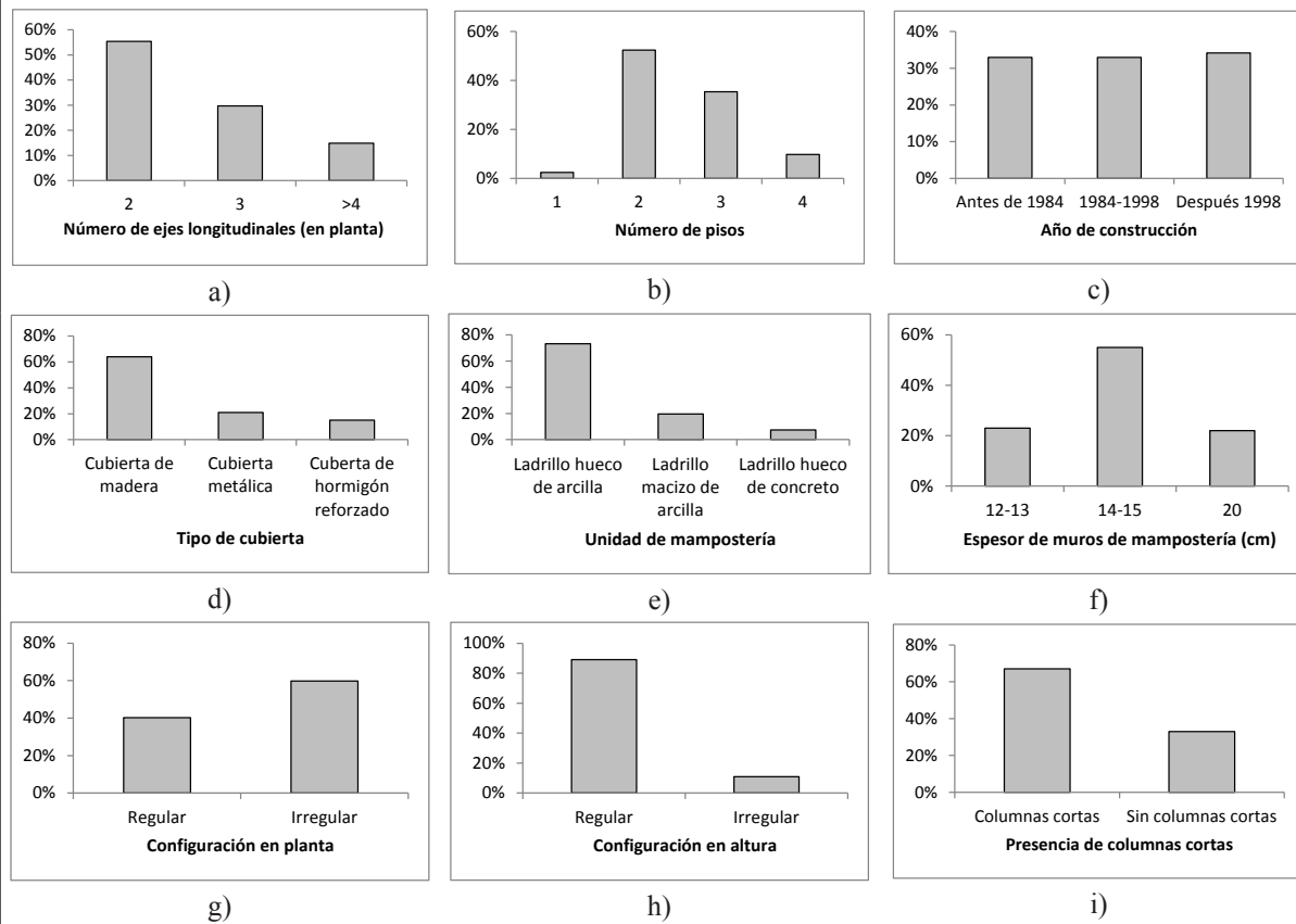
Figura 3. Configuración estructural típica de las escuelas
