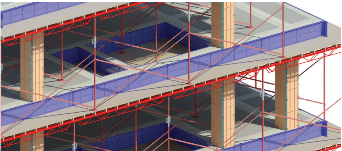
Figura 6. Sección del Modelo BIM 3D.
