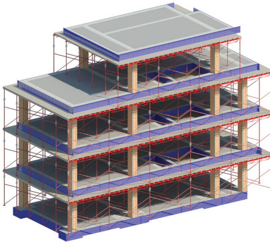
Figura 5. Modelo BIM 3D.
