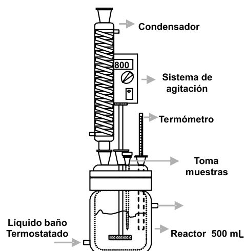
Figura 1. Sistema de reacción por lotes utilizado en los ensayos de laboratorio
