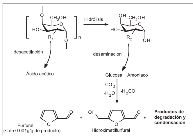
Figura 7. Esquema de rutas de reacción para conversión hidrotérmica de sustancias pécicas y quitina. Fuente: adaptado de Luijckx, 1993; Quitain, 2001; Miyazawa, 2004 y Srokol, 2004. R_1 = -NH-COCH_3 (para quitina), -COOH (para pectina) R_2 = -NH_2 (para quitina), -OH (para pectina)
