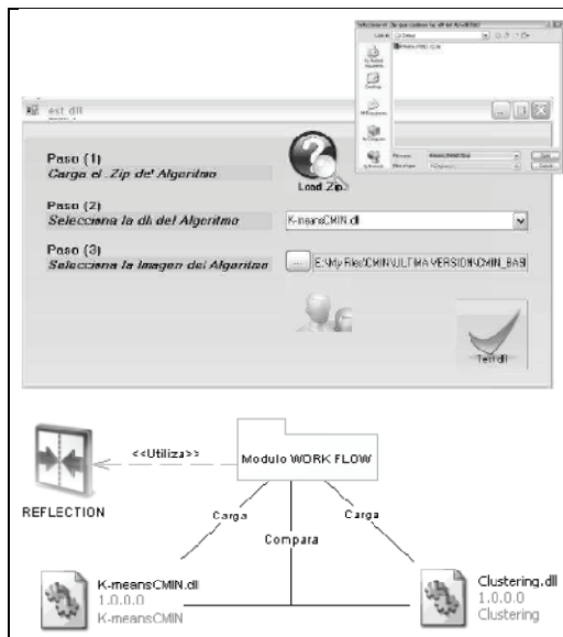
Figura 10. Adición de un nuevo algoritmo (izquierda) y validación de la DLL (derecha) en CMIN
