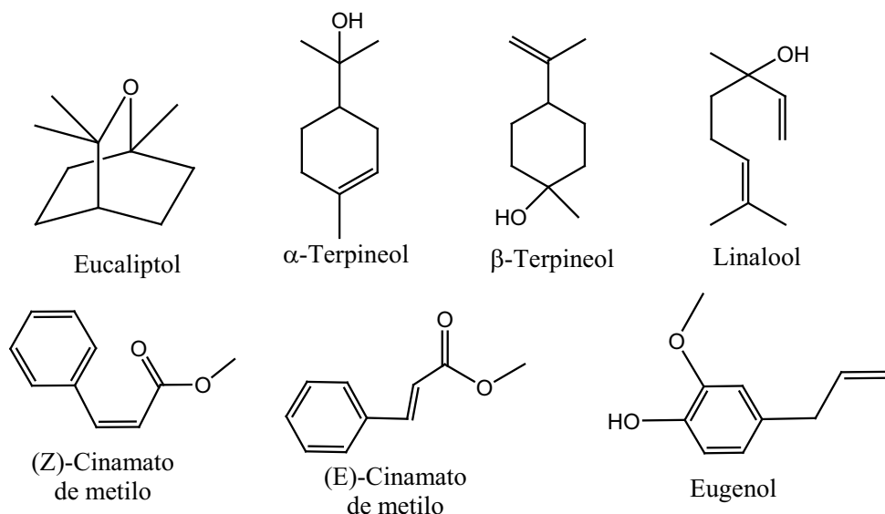
Figura 1. Estructura química de los componentes mayoritarios de los aceites esenciales de O. basilicum L. var cinammom , O. anisatum , O. purpurescens , O. album , O. thyrsoiflorum , O. cf. gratissimum .
