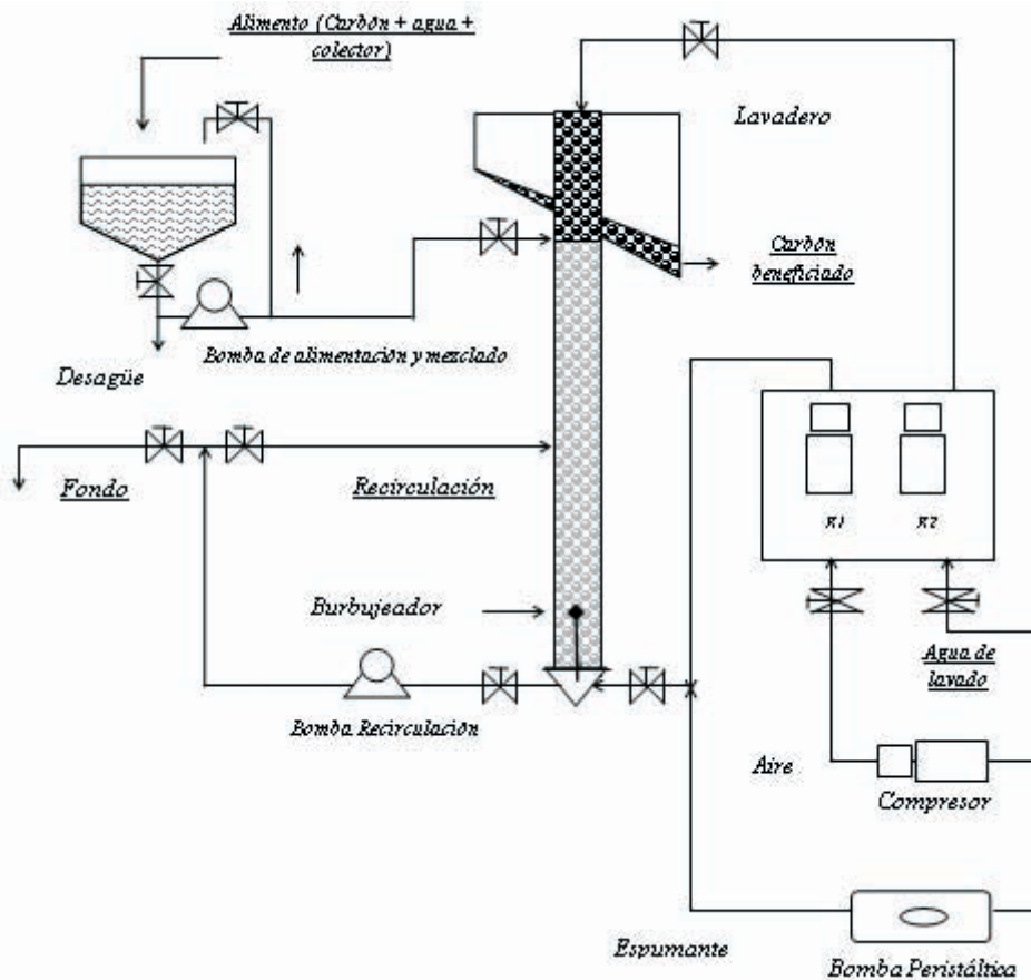
Figura 1 Diagrama de la columna de flotación a escala piloto. R1:Rótmetro de aire, R2:Rótmetro de agua
