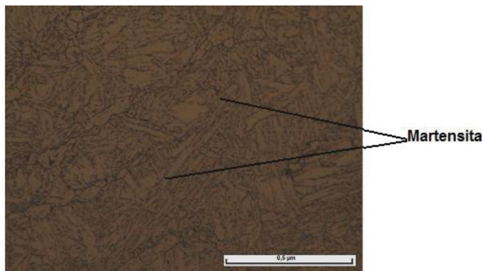
Figura 15. Micrografía en estado de entrega del acero ASTM A335 P92. 1000x.
