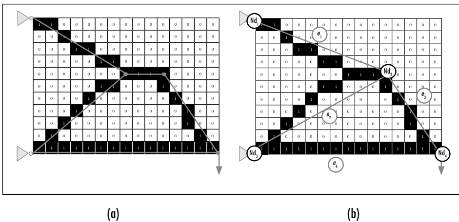
Figura 8. Resultado obtenido luego del colapso (a) a nodos de carga y de frontera y (b) entre nodos cercanos
