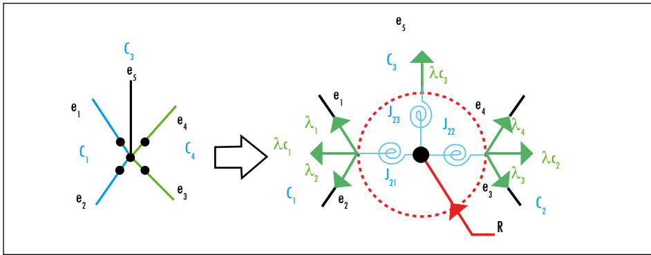
Figura 12. Proceso de expansión de nodos para el análisis estructural
