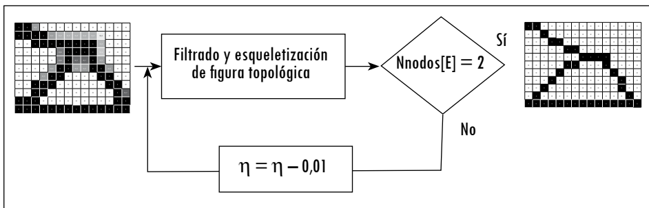
Figura 7. Proceso de evaluación de \eta
