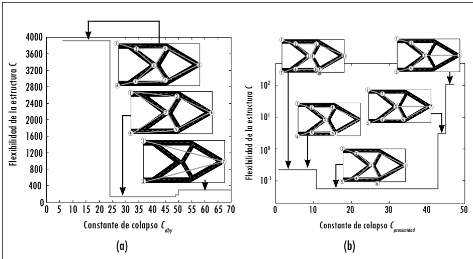
Figura 17. (a) Análisis de sensibilidad de C_{bdy} y (b) Análisis de sensibilidad de C_{proximidad} para el caso I
