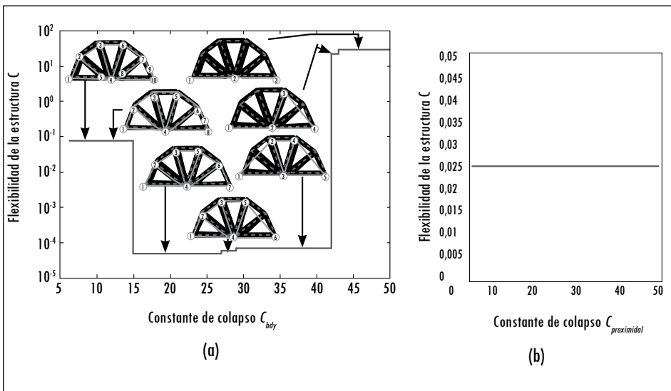
Figura 18. (a) Análisis de sensibilidad de C_{bdy} y (b) Análisis de sensibilidad de C_{proximidad} para el caso II
