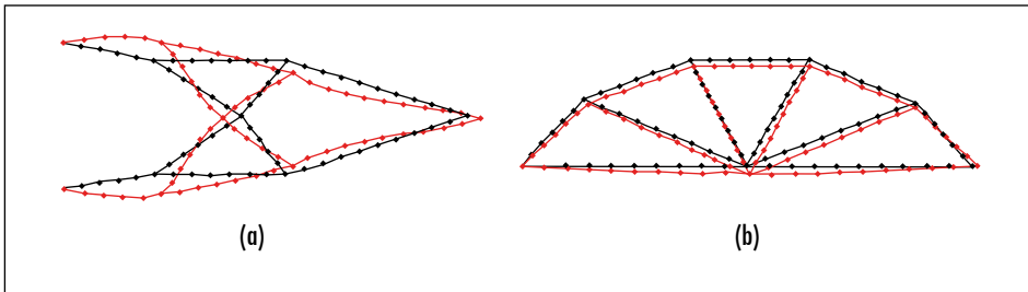
Figura 22. Estructuras deformadas con J_{ij} = \infty (unión rígida). Escala de deformación: (a) 1:50 y (b) 1:20.000
