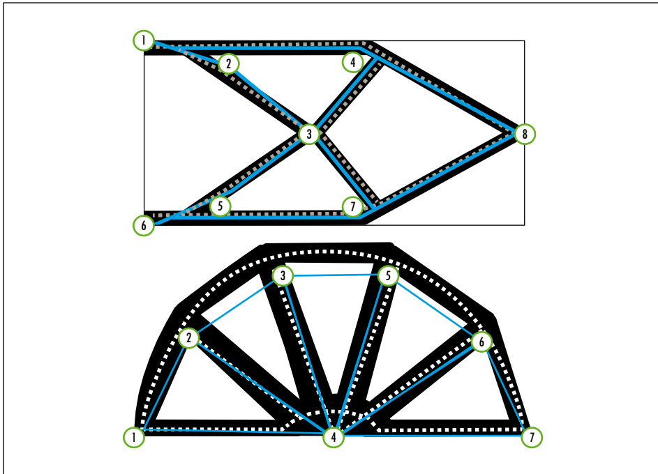
Figura 19. Aplicación de identificación de nodos y elementos para C_{bdy} = 0,15 y C_{proximidad} = 0,15 en los casos I y II respectivamente
