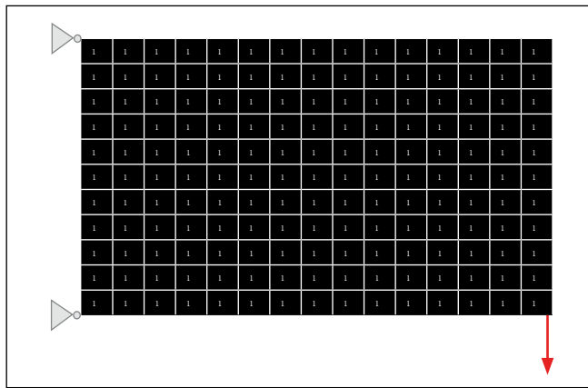
Figura 2. Dominio de diseño ( nelx = 15 y nely = 11)
