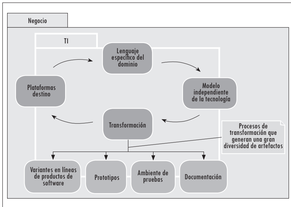
Figura 2. Consideraciones para la transformación de modelos en MDSD
