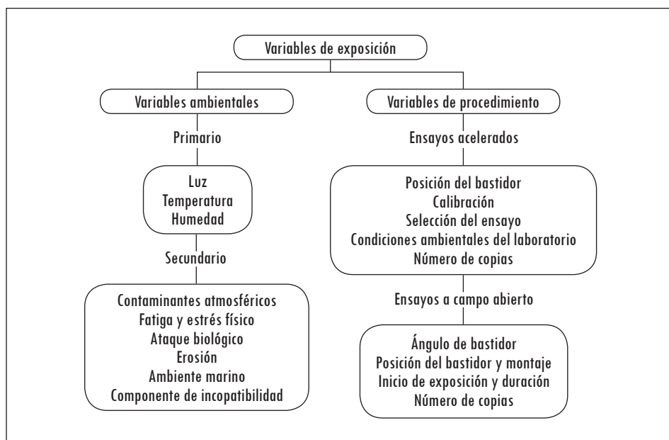
Figura 1. Variables importantes en ensayos de exposición
