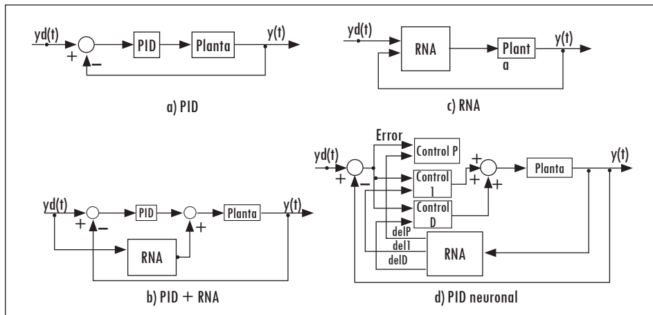
Figura 2. Estrategias de control: a) PID, b) PID + RNA, c) RNA y d) PID neuronal
