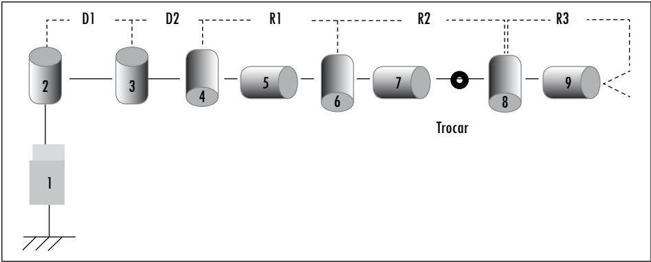
Figura 1. Esquema robot LapBot
