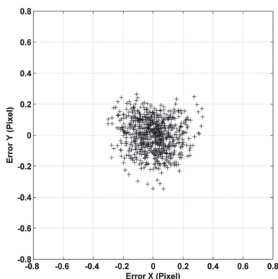
Fig 10. ERROR DE REPROYECCIÓN DEL PATRÓN AJEDREZADO
