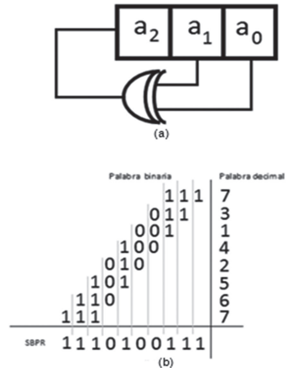
Fig. 2. (a) RETROALIMENTACIÓN DE DESPLAZAMIENTO LINEAL; (b) SECUENCIA BINARIA PSEUDO ALEATORIA
