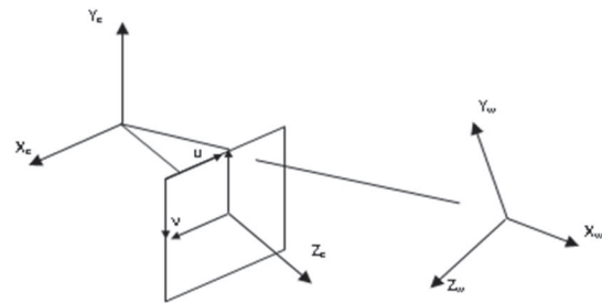
Fig. 6. MODELO “PINHOLE” PARA LA CÁMARA
