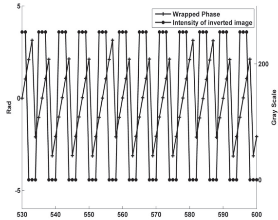
Fig. 5. FASE DISCONTINUA E INTENSIDAD DE LA IMAGEN INVERTIDA A LO LARGO DE LA DIRECCIÓN A – A' EN LA FIG. 3(a)
