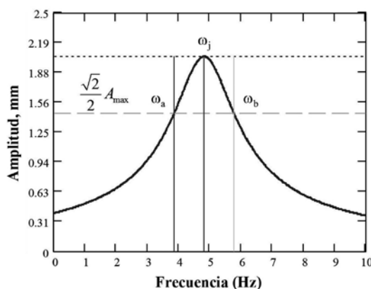
Fig. 1. MÉTODO DE LA MEDIA POTENCIA PARA DETERMINAR EL FACTOR DE PÉRDIDA \eta_j
