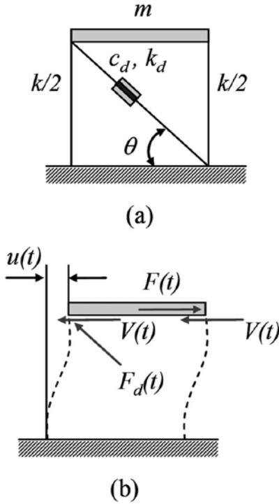
Fig. 3. (a) MODELO DE UN PÓRICO CON AMORTIGUADOR VISCOELÁSTICO. (b) DIAGRAMA DE CUERPO LIBRE
