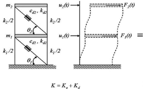
Fig. 4. PÓRICO DE DOS PISOS CON AMORTIGUADOR VISCOELÁSTICO
