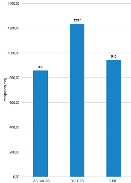
Fig. 6. PRECIPITACIÓN MENSUAL MULTIANUAL
