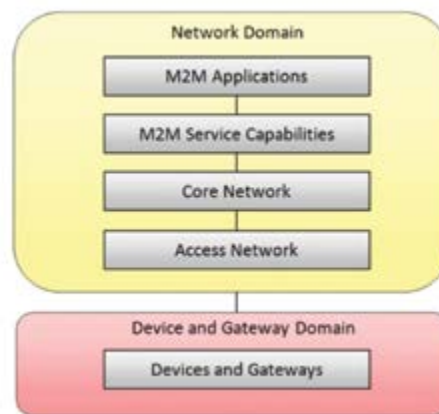
Fig. 1. DOMINIOS DE LA ARQUITECTURA FUNCIONAL M2M DE ETSI [14]
