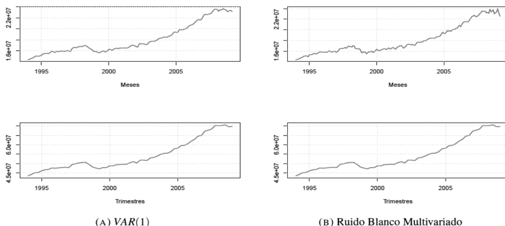
Gráfico 2. Serie estimadas del PIB suponiendo que los errores de alta frecuencia siguen un proceso ruido blanco multivariado y un VAR (1)
