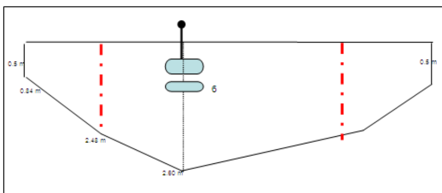
FIGURA 3. Perfil del lago 2
