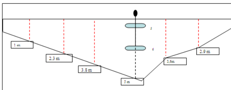
Figura 2. Perfil del lago 1
