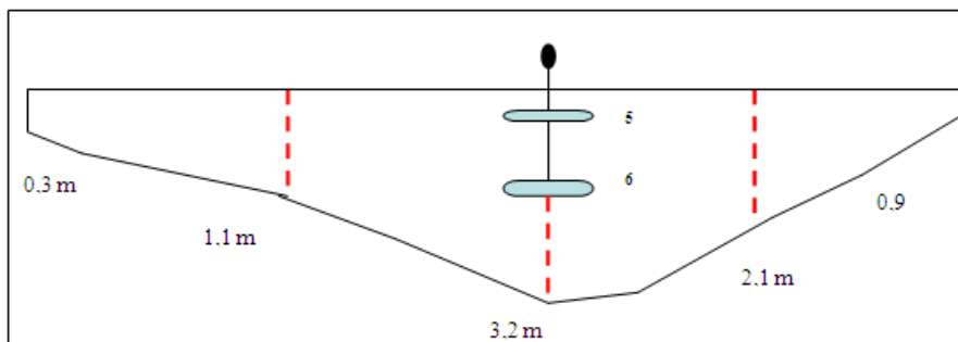
FIGURA 4. Perfil del lago 3
