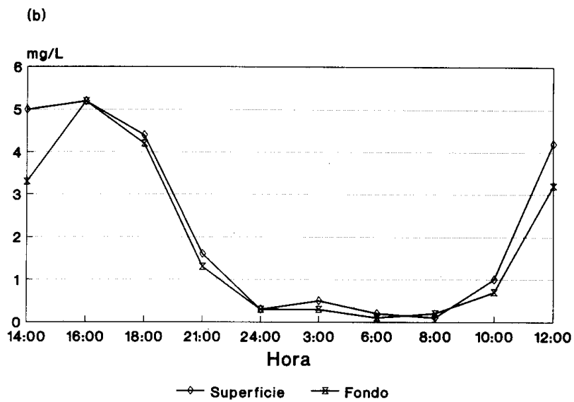
Figura 3. Curvas de oxígeno disuelto obtenidas en agosto 30-31/94 en Caño Grande (a) y El Morro (b). Para aguas de igual densidad, los valores de saturación de oxígeno están entre 5.3 y 5.9 mg/l para (a) y entre 5.0 y 5.5 mg/l para (b).
