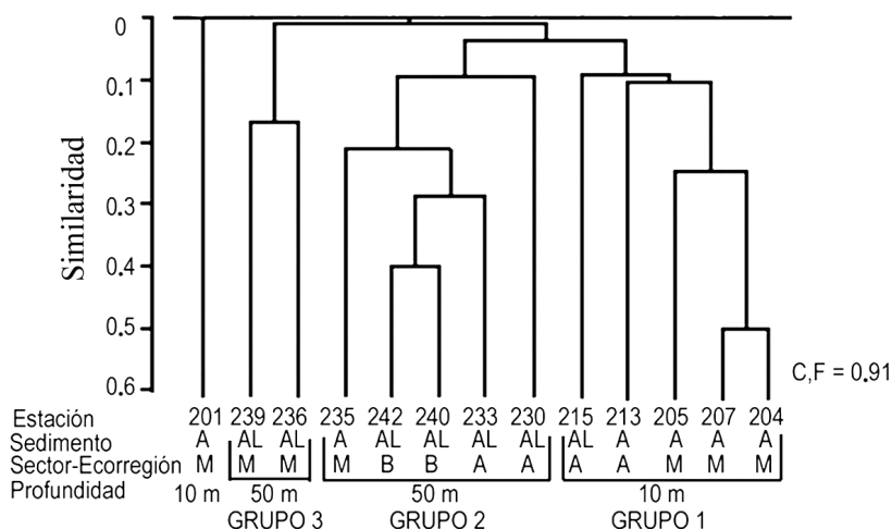
Figura 2. Análisis clúster de las estaciones donde aparecieron esponjas en La Guajira, basado en la presencia-ausencia de especies. Los valores de similaridad fueron calculados usando el coeficiente de Jaccard, 0.6 indica la mayor similaridad. Bajo el número de cada estación se muestra el sedimento dominante (A: arena. AL: arena-lodosa), el sector geográfico y ecorregión donde se ubica (a: alto. m: medio. Ecorregión La Guajira. b: bajo. Ecorregión Palomino), y la profundidad (10 ó 50 m). Coeficiente cofenético de correlación (C,F) = 0.91.
