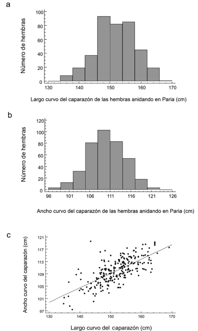
Figura 4. Medidas del caparazón de las hembras (longitud curva del caparazón) anidando en la península de Paria (playas Cipara y Querepare). (a) LCC ( \bar{X} \pm DE )= 151.78 \pm 6.20 cm, (b) ACC ( \bar{X} \pm DE )= 110.03 \pm 4.42 cm y (c) relación ancho vs largo del caparazón ( ACC = 39.205 + 0.46607 \cdot LCC , R^2 = 49.6 , F_{1,232} = 228.3 , p < 0.0001 ).
