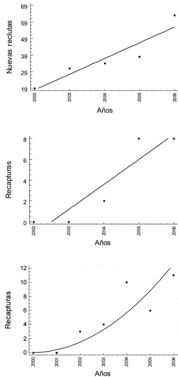
Figura 3. (a) Número de nuevas reclutas anuales para Querepare ( r= 0.929 , p= 0.022 , hembras nuevas = -19001.0+9.5\cdot\text{año} ), (b) número de reemigrantes ( r= 0.926 , p= 0.024 , recapturadas= -4806.0+2.4\cdot\text{año} ) y (c) número de reemigrantes para Cipara ( r= 0.923 , p= 0.003 ), recapturadas = (-1162.7+0.6\cdot\text{año})^2 . El número de hembras nuevas para Cipara no se ha incrementado de manera significativa.
