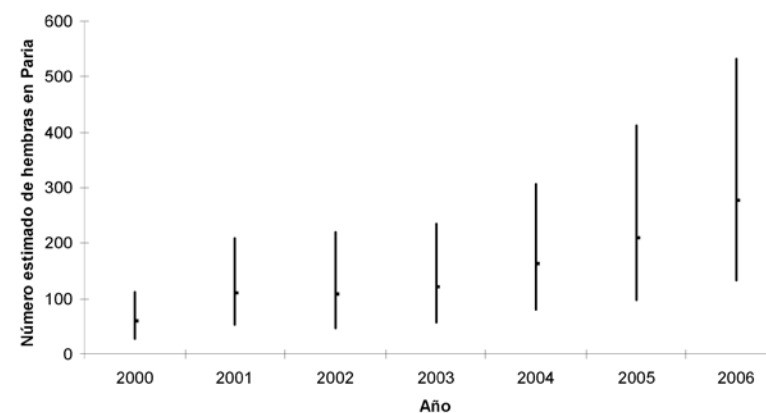
Figura 6. Estimados del número de hembras anidando en la totalidad de las playas de Paria entre 2000 y 2006. La barra vertical indica los límites de confianza y la horizontal la media de la estimación.
