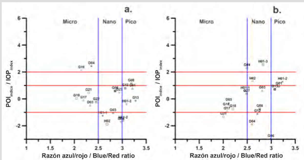
Figura 2. Relación del Índice de IOP_{Index} con la estructura de tamaño para identificar florecimientos en Estaciones: a. superficiales 2017, b. en el MPC en 2017.
