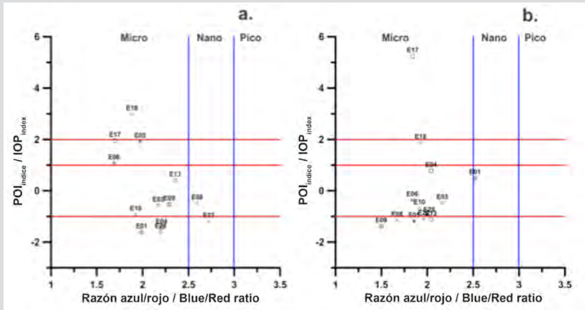
Figura 5. Relación del Índice de POI índice con la estructura de tamaño para identificar florecimientos en Estaciones: a. superficiales 2018, b. en el MPC en 2018.
