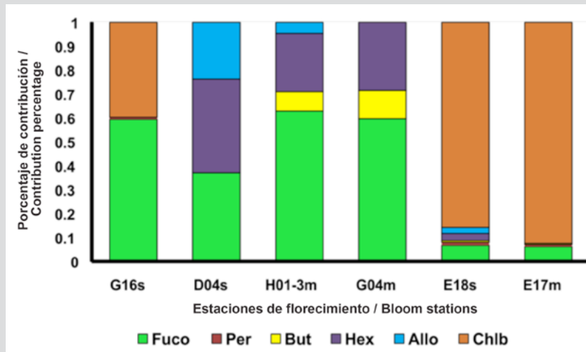
Figura 4. Porcentaje de contribución de los pigmentos fucoxantina (Fuco), peridinina (Per), butaniloixifucoxantina (But), hexanoiloxifucoxantina (Hex), alloxantina (Allo), clorofila b (Chl-b), en las estaciones en florecimiento donde: 2017 en superficie (G16, D04) y MPC (H01-3, G04); 2018 en superficie (E18) y en MPC (E17).
