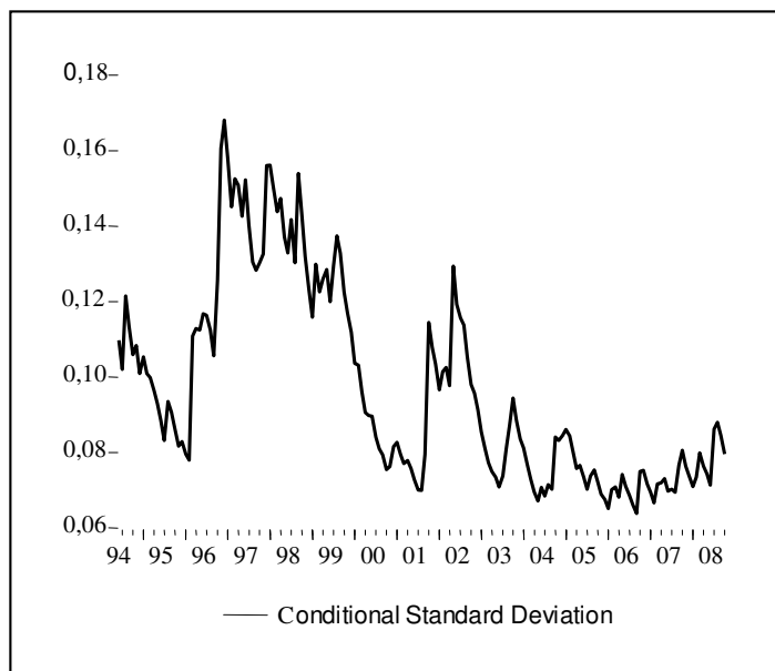
Gráfico 6 Desviación estándar de las expectativas Modelo Garch(1,1)
