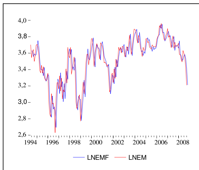
Gráfico 5 Ajuste ARMA de las expectativas empresariales en la EOIC
