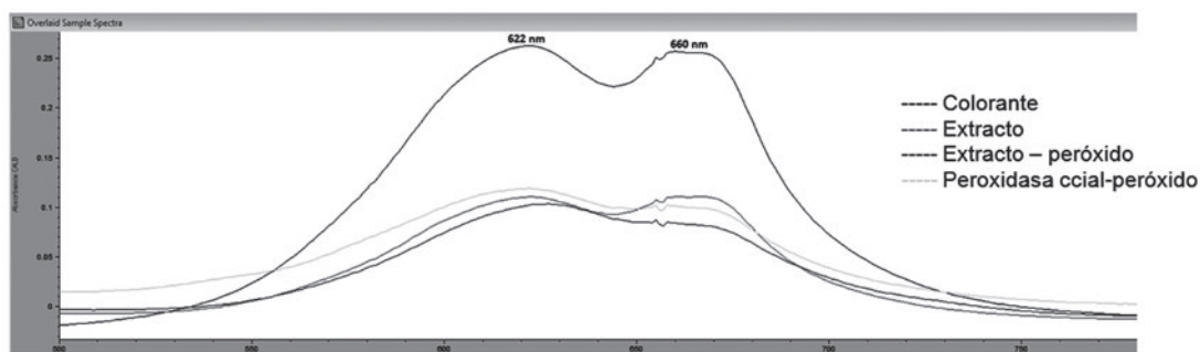
Figura 6. Espectro de absorbancias del colorante Azul Reactivo 2I con un tiempo de residencia t = 0 min
