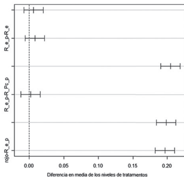
Figura 5. Intervalos de confianza HSD para el colorante Rojo reactivo 14I
