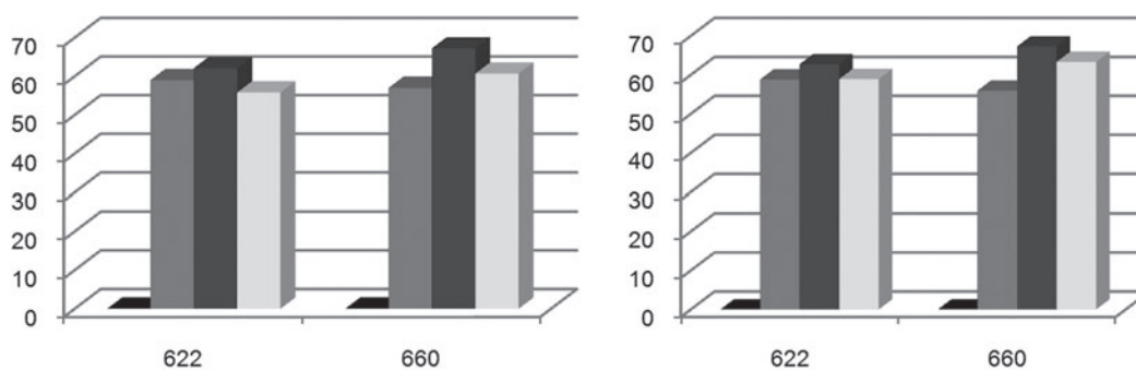
Figura 7. Porcentajes de decoloración del Azul reactivo 21 a tiempos de residencia 0 y 10 minutos respectivamente
