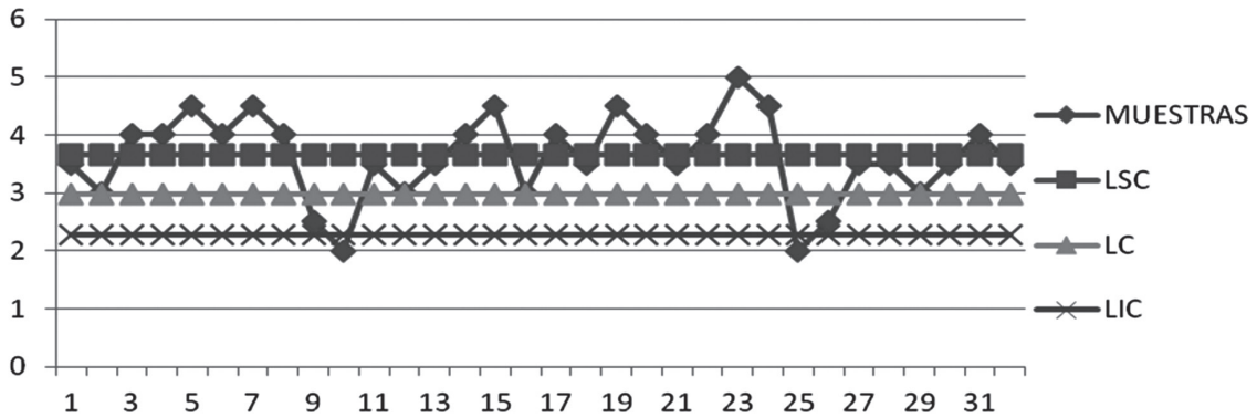
Figura 2. Gráfico de control para los datos antes de la mejora
