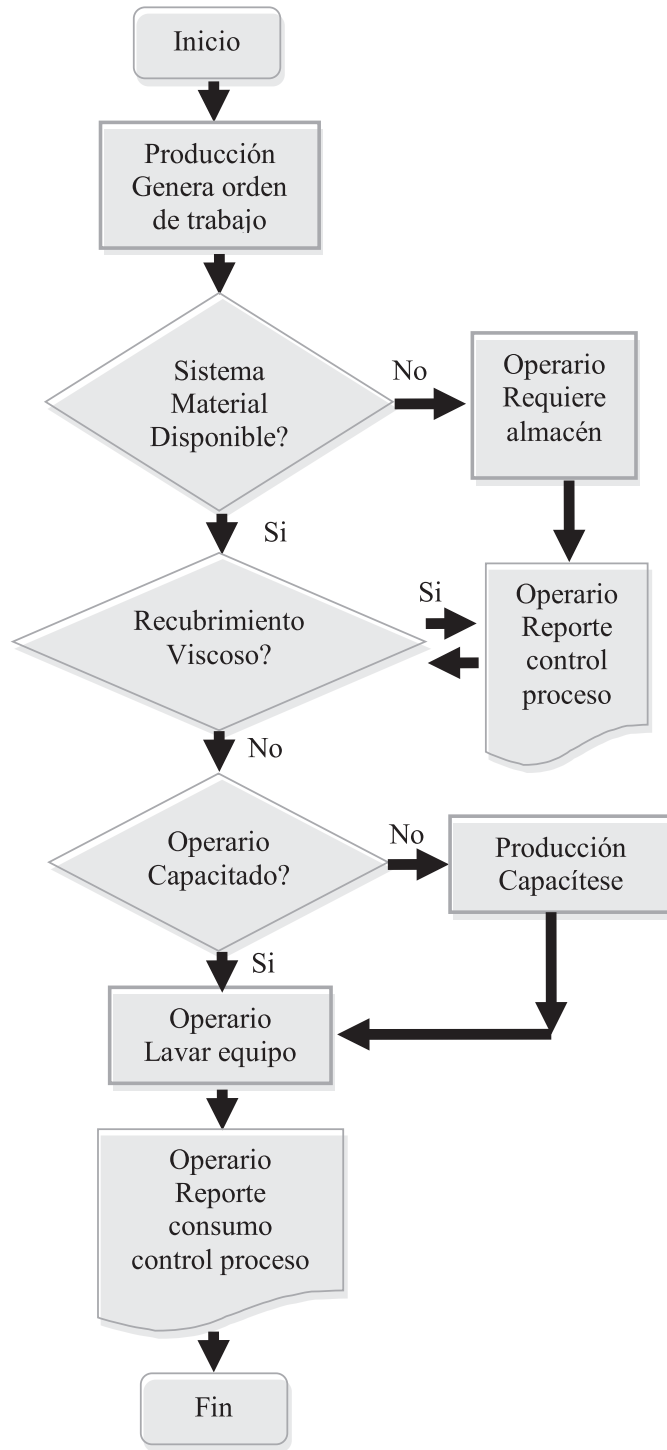
Figura 1. Flujograma para el consumo de disolvente
