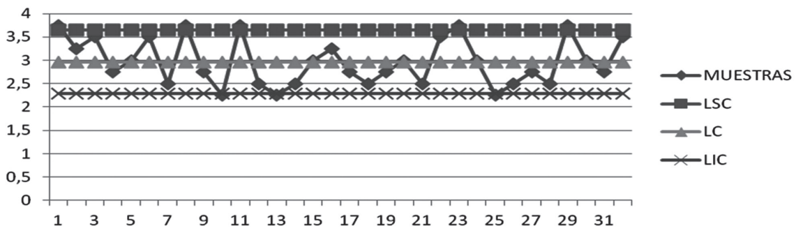
Figura 3. Gráfico de control para los datos después de la mejora
