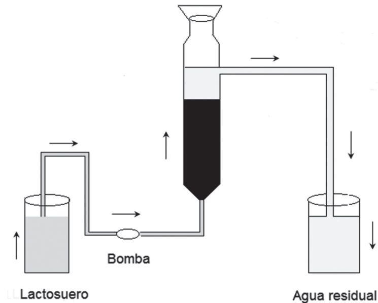
Figura 1. Diagrama de reactor UASB tratando lactosuero
