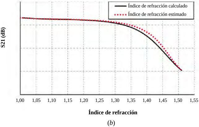
Figura 5. Estimación del índice de refracción de tres materiales utilizando el metamaterial desarrollado, (a) por variación de la f_c y (b) por variación de S_{21} .
