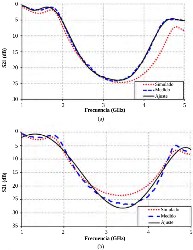
Figura 4. Parámetro de dispersión Vs. frecuencia (dato ajustado). (a) Agua destilada y (b) aceite de inmersión de tipo F, dentro de la estructura EBG.
