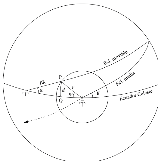
Figura 3. Modelo general de la trepidación. El fenómeno de precesión propiamente dicho hace que el punto vernal medio ( \Upsilon ) avance a una velocidad uniforme en la dirección de la flecha segmentada. La trepidación propiamente dicha es la distancia \Delta\lambda ( \Upsilon -P), que puede ser positiva o negativa.
