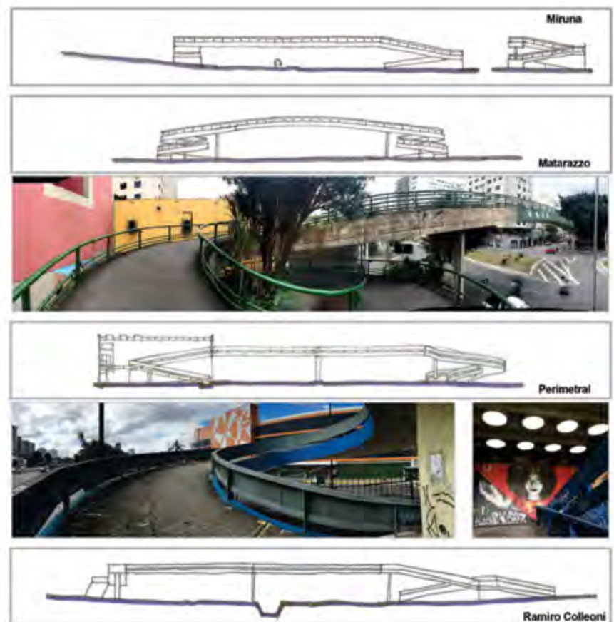
■ Figura 8. Dibujos y fotografías de rampas en pasarelas urbanas diseñadas por Vilanova Artigas. Miruna y Matarazzo (con foto) en São Paulo. Perimetral (con foto) y Ramiro Colleoni en Santo André. Fuente: elaboración propia (2019).
