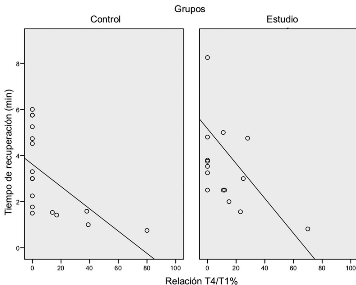
Figura 3. Correlación lineal, dispersión de puntos de datos, tiempo de recuperación y relación T4/T1. R^2 lineal = 0,339 para el grupo control y 0,212 para el grupo de estudio. Min = minutos.
