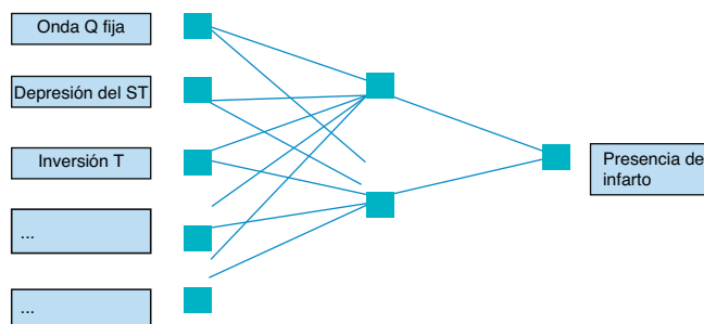
Figura 1 Ejemplo de una red neuronal con 5 neuronas (variables) de entrada, 2 neuronas en la capa oculta y una neurona de salida.
