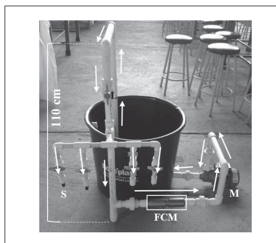
Figura 1. Circuito de recirculación de agua con magnetizadores. L: llave de paso de agua, S: salida del ATM hacia el sistema de riego, FCM: fuente de campo magnético, M: motobomba eléctrica, las flechas indican el flujo de recirculación de entrada/salida.
