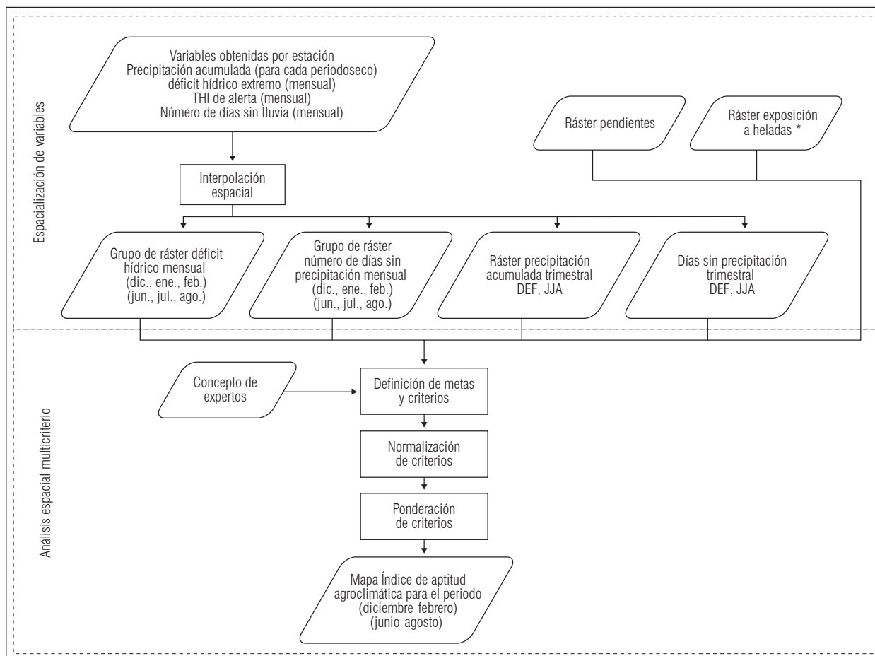
Figura 2. Diagrama de flujo del análisis espacial multicriterio para la obtención del IAC durante los períodos DEF y JJA. El criterio referente a exposición a heladas solo se consideró en el período seco de DEF (* raster normalizado).
