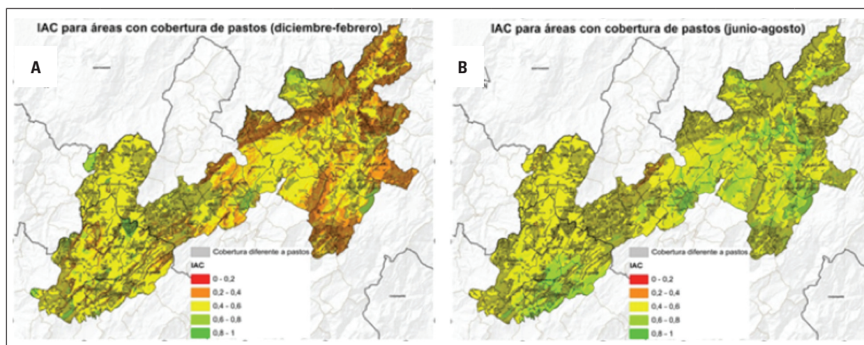
Figura 5. Distribución espacial del IAC para los períodos secos DEF (A) y JJA (B).
