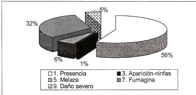
Figura 3. Porcentajes de la estimación visual a nivel de daño de T. vaporariorum en hojas y/o folíolos de tabaco y fríjol en la provincia de García Rovira (Santander). 1. Presencia de adultos o huevos; 3. Aparición de las primeras ninfas en el tercio inferior de la planta; 5. Gotas de melaza (brillo en hojas, dos tercios de la planta con melaza); 7. Aparición de fumagina, daño severo y 9. Hojas y vainas cubiertas con fumagina, daño muy severo.
