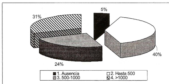
Figura 2. Porcentajes de la estimación visual a nivel de huevos, ninfas y adultos de T. vaporariorum en hojas y/o folíolos de tabaco y fríjol en la provincia de García Rovira (Santander). 1. Ausencia de inmaduros y/o adultos; 2. Hasta 500 inmaduros o adultos por hoja; 3. De 500 a 1.000 individuos por hoja y 4. Más de 1.000 individuos por hoja.
