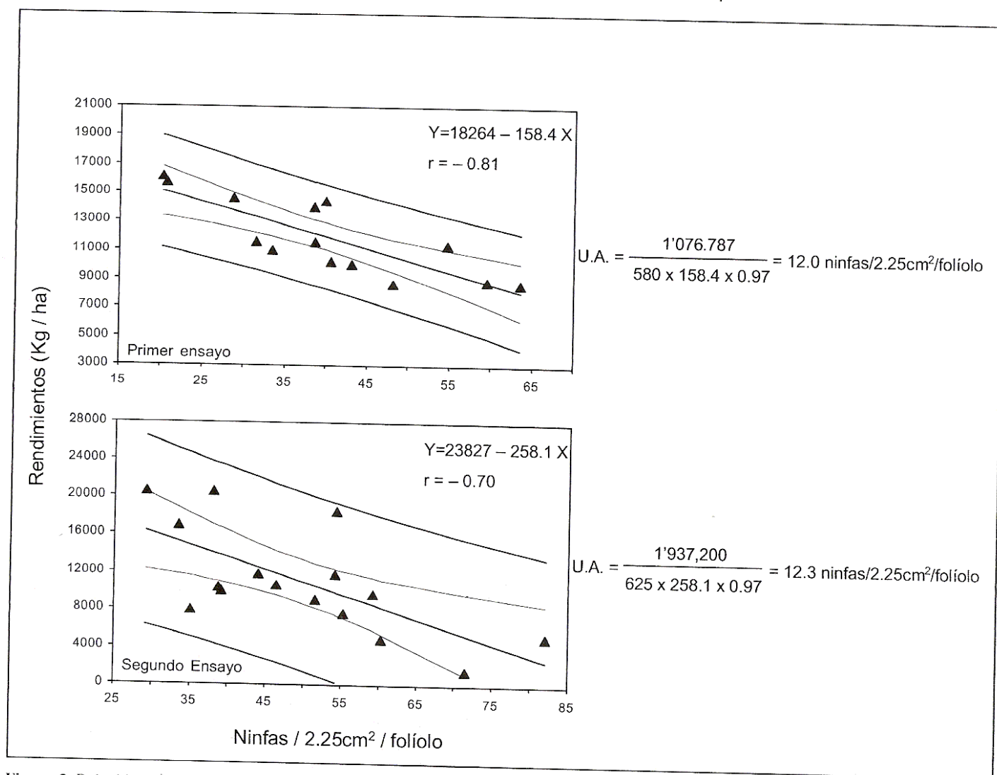
Figura 2. Relación entre los niveles de infestación de ninfas de primer instar de Trialeurodes vaporariorum y los rendimientos de habichuela. Intervalos de confianza al 95%. Cálculo del umbral de acción en dos ensayos.
