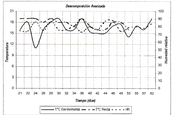
Figura 2. Curvas de temperatura ambiental, temperatura rectal y humedad relativa para el estado de descomposición avanzada.
