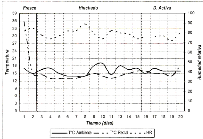
Figura 1. Curvas de temperatura ambiental, temperatura rectal y humedad relativa para los estados de descomposición fresco, hinchado y de descomposición activa.
