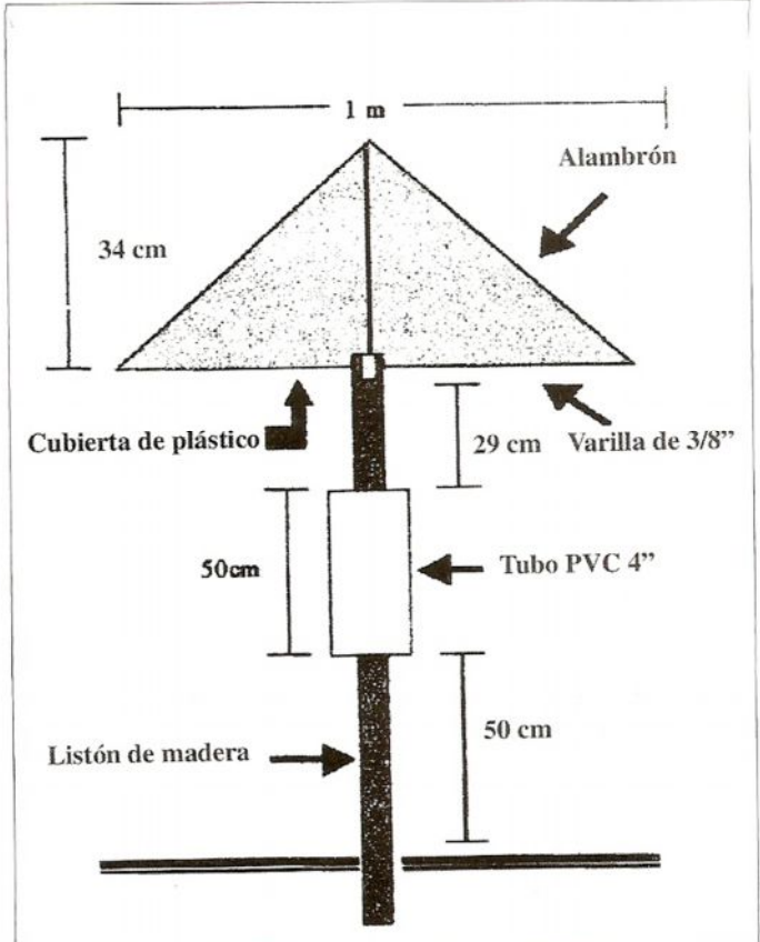
Figura 2. Esquema de la trampa ubicada en los diferentes cultivos de flores (Tomado de ICA, ASOCOLFLORES, 2000).
