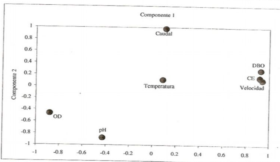
Figura 2. Ordenación de ACP de los parámetros fisicoquímicos del río Rímac, Lima, Perú.
