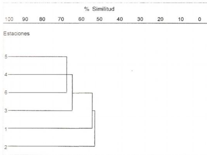
Figura 3. Análisis cualitativo de similitud empleando el Índice de Sørensen para las estaciones de muestreo en el río Rímac. 1. Puente Graña; 2. Canal Huatica; 3. Puente Trujillo; 4. Puente del Ejército; 5. Puente Faucett; 6. Puente Gambeta.
