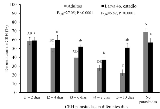
Figura 2. Porcentaje de depredación de C. montrouzieri , adulto y larva de cuarto estadio en pruebas de no elección sobre CRH parasitadas por A. kamali de 2, 4, 6, 8 y 10 días y no parasitadas. Las letras mayúsculas se refieren al análisis de comparación de medias en los porcentajes de depredación del adulto y las minúsculas el de porcentaje de depredación de larvas de cuarto estadio.
