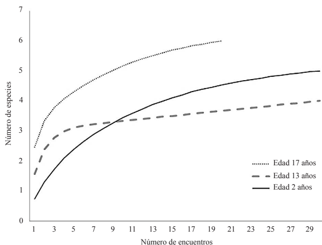
Figura 2. Curvas de acumulación de especies de termitas por edad de plantación. Estimador Chao 2.
