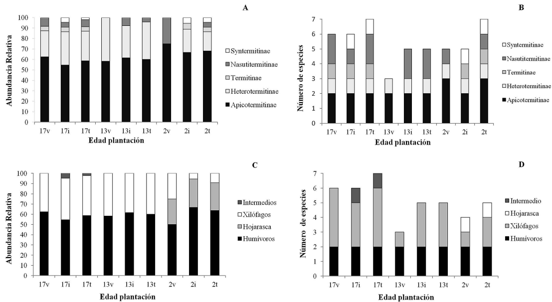
Figura 1. Abundancia y riqueza de especies en diferentes edades de plantación de caucho. A. Abundancia relativa por subfamilia. B. número de especies por subfamilia. C. Abundancia relativa por grupo trófico. D. número de especies por grupo trófico. i: temporada de lluvias, v: temporada seca, t: total temporada de lluvias mas temporada seca.
