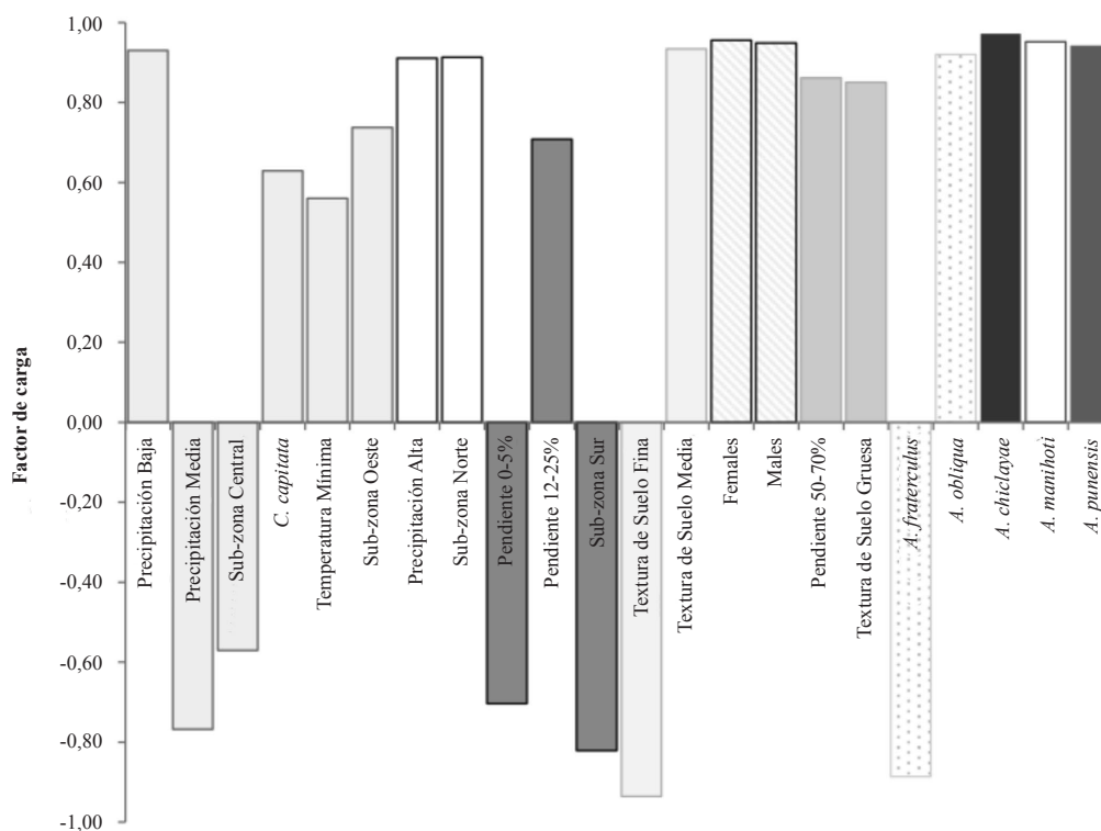
Figura 2. Representación del factor carga (entre 0 and \pm 1 ) por variable de acuerdo a la matriz rotada de Varimax, para la interpretación del análisis de componentes principales (PCA), en la península de Santa Elena, Ecuador.
