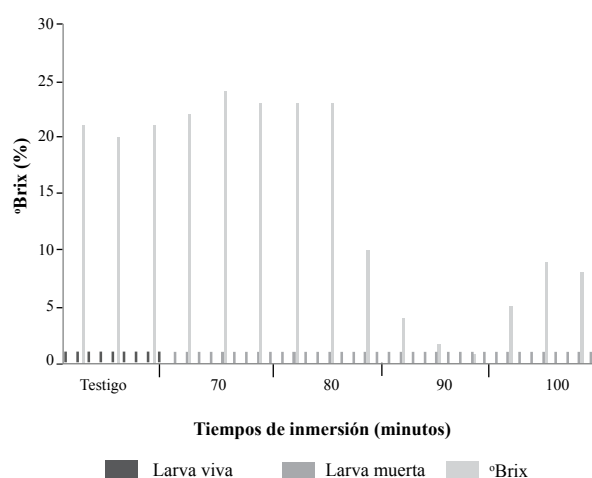
Figura 2. °Brix de frutos de guayaba en tratamiento hidrotérmico a 65 °C con larvas de C. dimidiatus .
