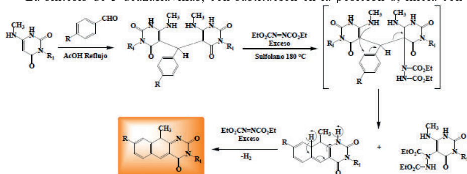
Esquema 6. Obtención de 5-deazaflavinas sustituidas en posición C-8 utilizando DAD.
