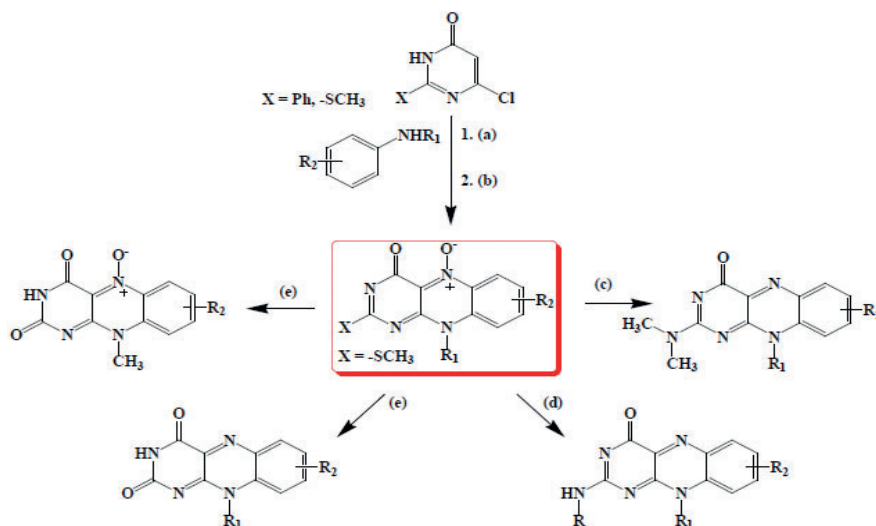
Esquema 16. Obtención de derivados tipo 2-deoxo-2-fenilflavin-5-óxidos. Reactivos y condiciones (a) En reacción de fusión con la apropiada amina, a temperatura entre 180–200° C, durante 0.5–5 h, en atmósfera de N 2 ; (b) reacción de nitrosación-ciclación con un exceso de NaNO 2 , AcOH, controlando la temperatura entre 10–15° C, durante 2–5 h; (c) Desoxigenación con 50 % acuoso NH(Me) 2 , en tubo sellado de acero, a temperaturas entre 160–165° C, durante 4 h; (d) sustitución con la apropiada amina, en n -BuOH a reflujo durante 15 min; (e) sustitución en presencia de HCl 5N, calentamiento a reflujo, durante 7–12 h.
