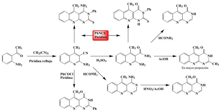
Esquema 12. Síntesis de 5-deazaflavinas a partir de 2-amino-4-metilquinolin-3-carbonitrilos.
