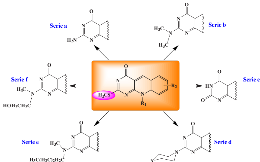
Esquema 17. Descripción general para la preparación de 10-alkil-2-amino-2-deoxo-5-deazaflavinas.
