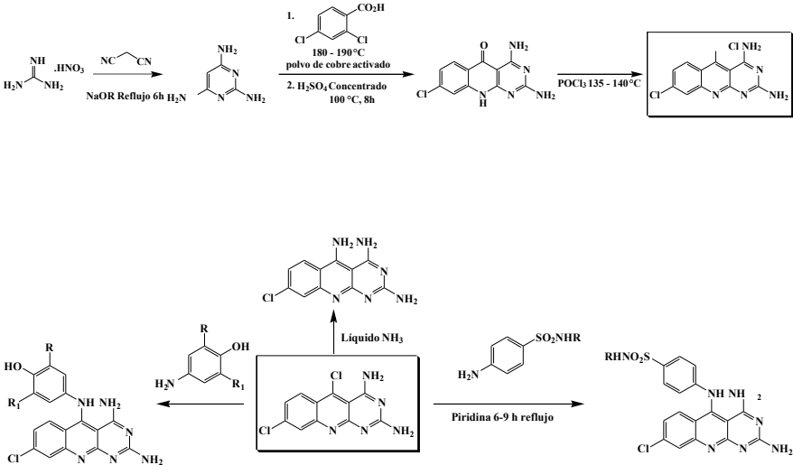
Esquema 11. Síntesis de derivados 5-deazaflavinas a partir de triaminopirimidina.
