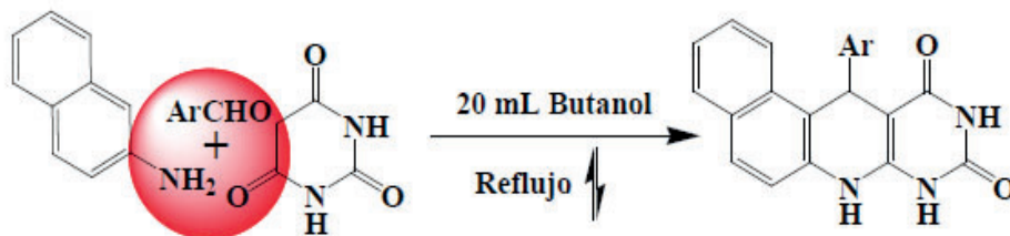
Esquema 4. Síntesis de pirimidoquinolinodionas.
