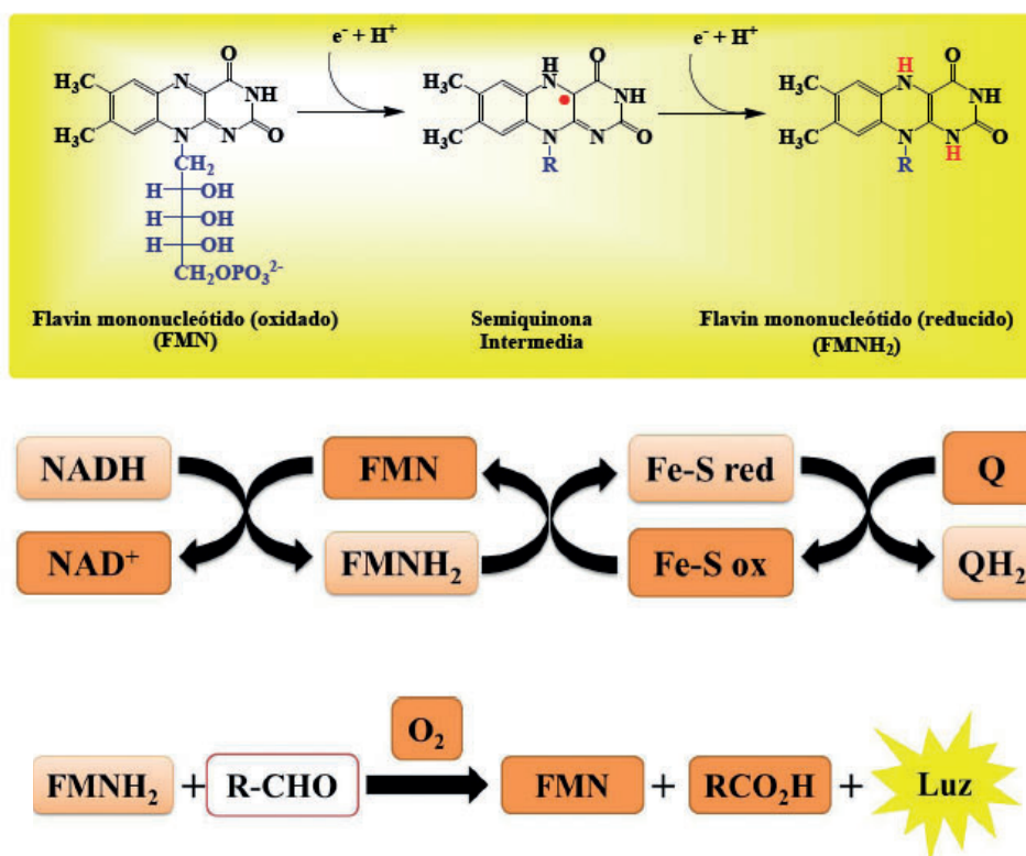
Esquema 1. Producción de luz mediante la oxidación catalítica en presencia de FMN-reductasa, dodecildehído y oxígeno.
