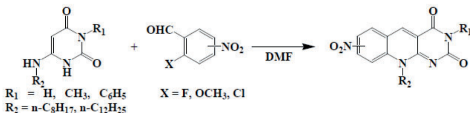
Esquema 7. Síntesis de 5-deazaflavinas nitro-sustituidas a partir de 6-aminouracilos en reacción con nitro-benzaldehídos.
