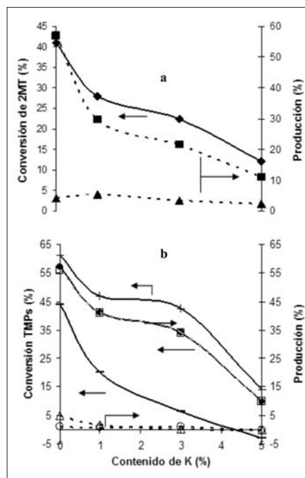
Figura 3. Efecto del contenido de potasio en los catalizadores CoMo/\gamma-Al_2O_3-K(x) sobre la conversión (líneas continuas) y la producción de cada uno de los compuestos (líneas punteadas). a): 2MT (◆), C5s (■), 2MTHT (▲). b): TM1P (+), TM2P (-), olefinas totales (●), iC8 (□), iC4 (△), isoTMP (○).
