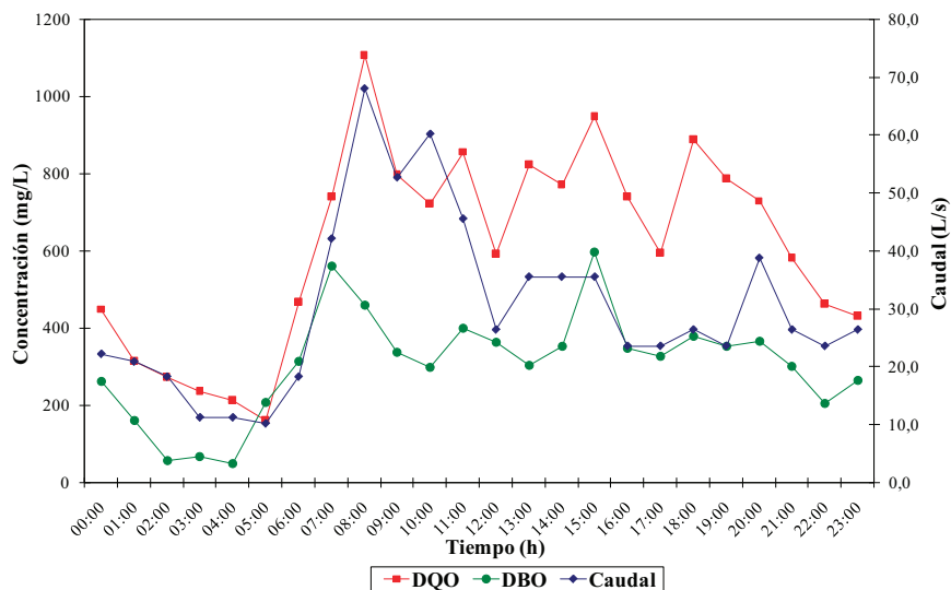
Gráfico 6. Variación del caudal, DQO y DBO afluentes a la ETAR a lo largo de 24h
